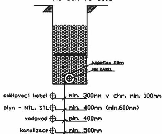
SOUBĚH S PODZEMNÍMI SÍTĚMI dle ČSN 73 6005
