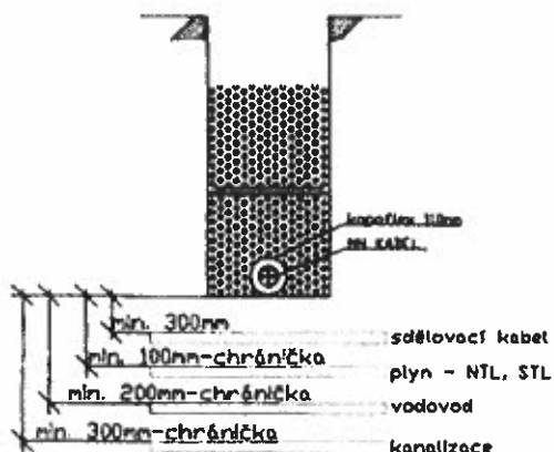
KŘÍŽENÍ S PODZEMNÍMI SÍTĚMI dle ČSN 73 6005
